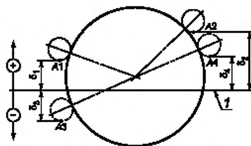
1 — линия номинального положения контрольных точек замков, наносимая на шаблон; \delta — измеряемое по вертикали отклонение замка от номинального положения; A1, A2 — контрольные точки первого торца; A3, A4 — контрольные точки второго торца; A1, A3 — контрольные точки первого замка; A2, A4 — контрольные точки второго замка
