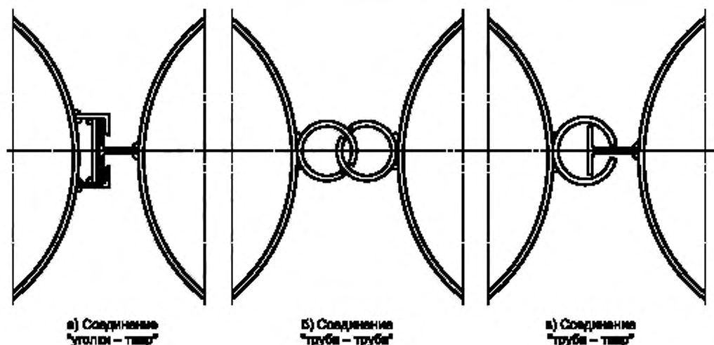
Рисунок 3 — Предпочтительные типы замковых соединений шпунтовых профилей
