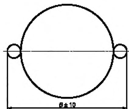
Рисунок 4 — Предельное отклонение ширины шпунтового профиля
