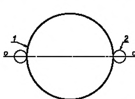
1 — труба; 2 — замок; O — O — ось шпунтовой стены
