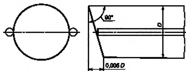
Рисунок 6 — Предельный перекося плоскости торца шпунтового профиля
